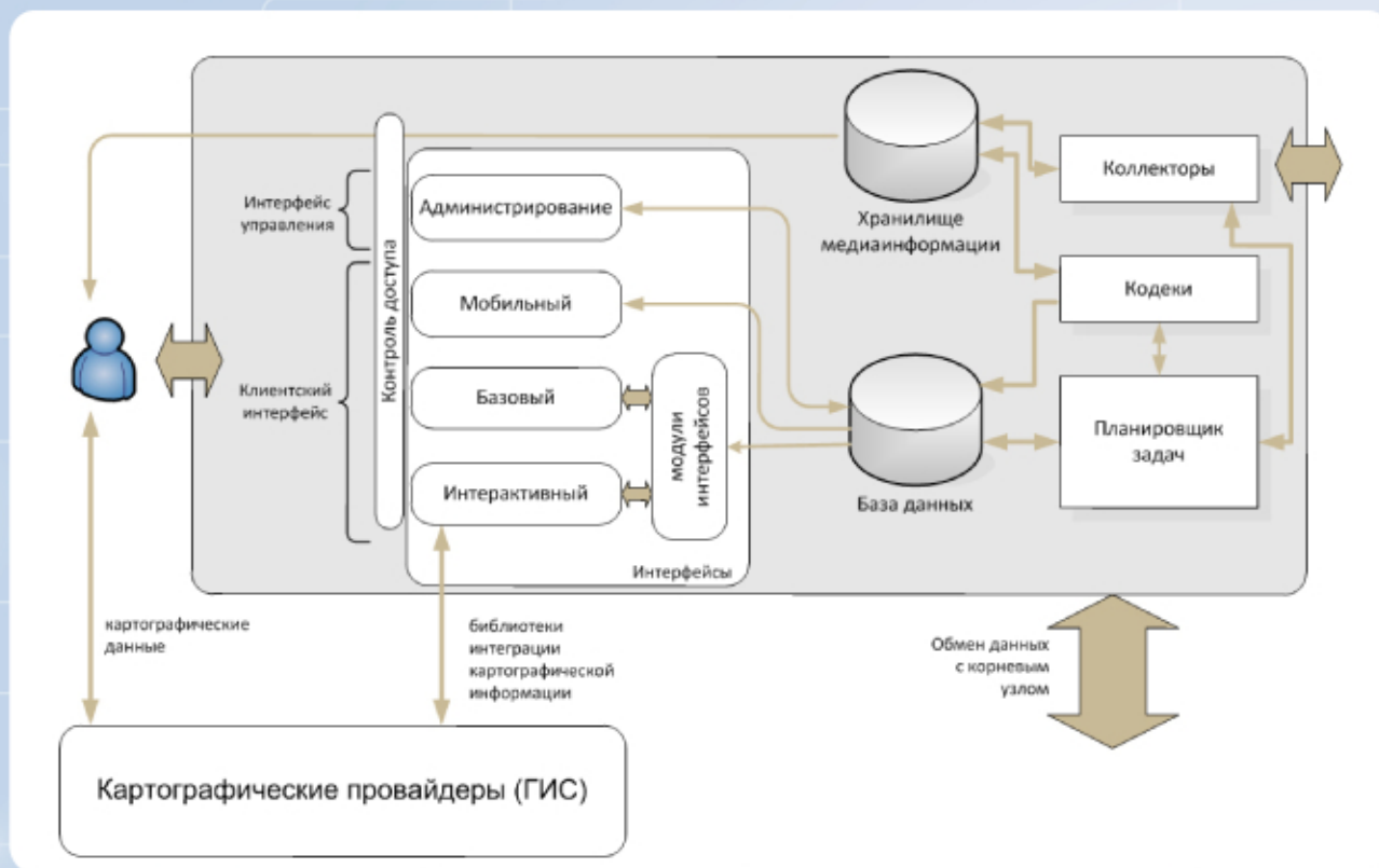
Функциональная схема центрального узла
